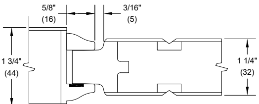
VG - V Groove
